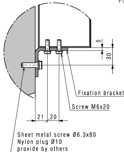
Détail B
