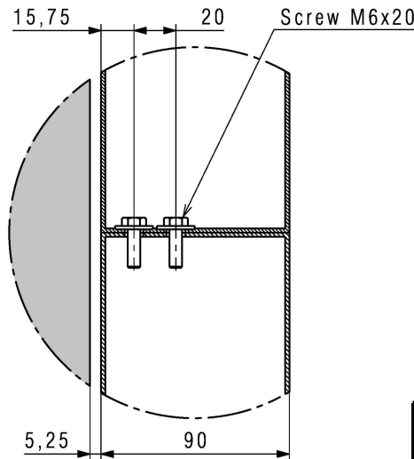
Détail C
