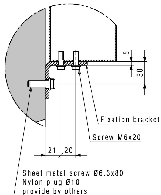
Détail B
