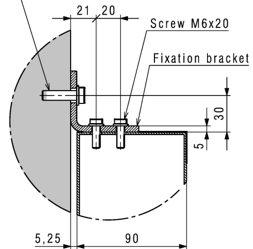
Détail B
