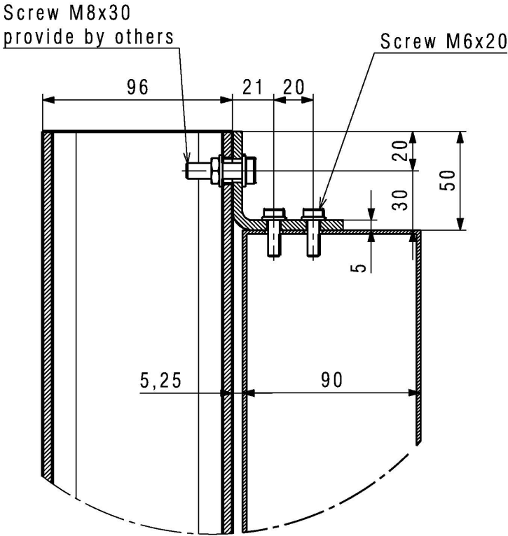
Détail A
