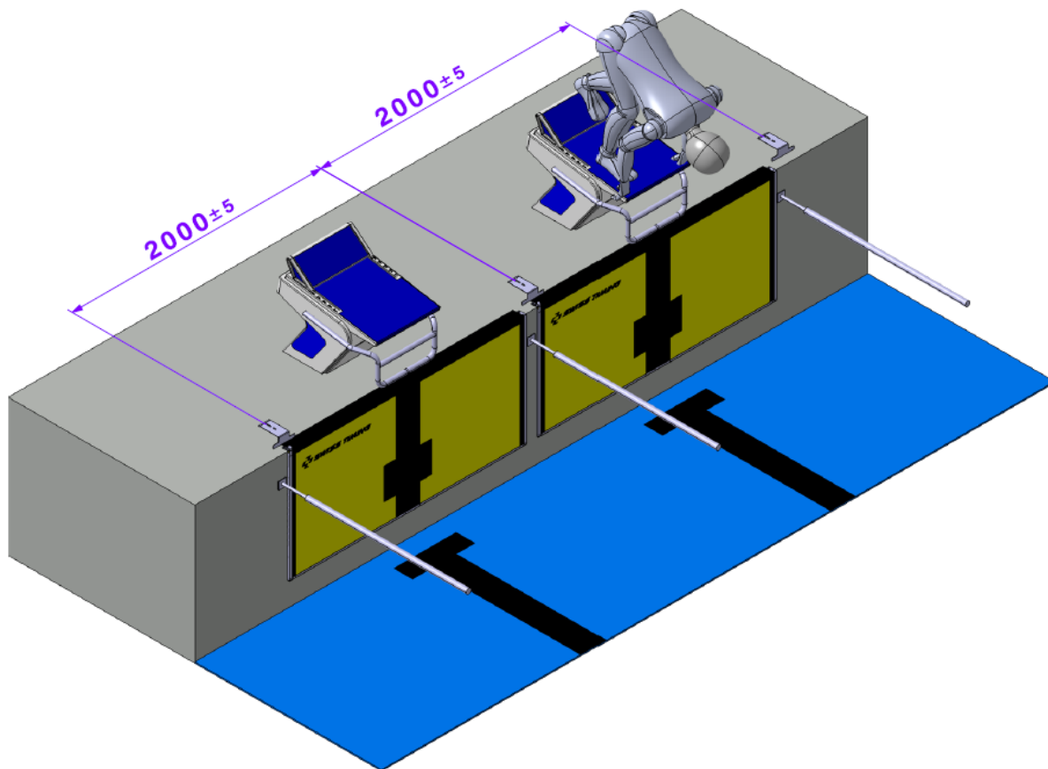
Abbildung 6 - Anschlagplatte 190x90 / Befestigung mit Haltewinkel
