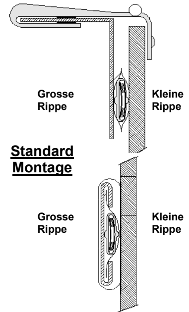
Abbildung 11 - Kontakt / Standard Montage
