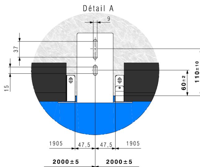
Abbildung 6 - Anschlagplatte 190x90 / Befestigung mit Haltewinkel
