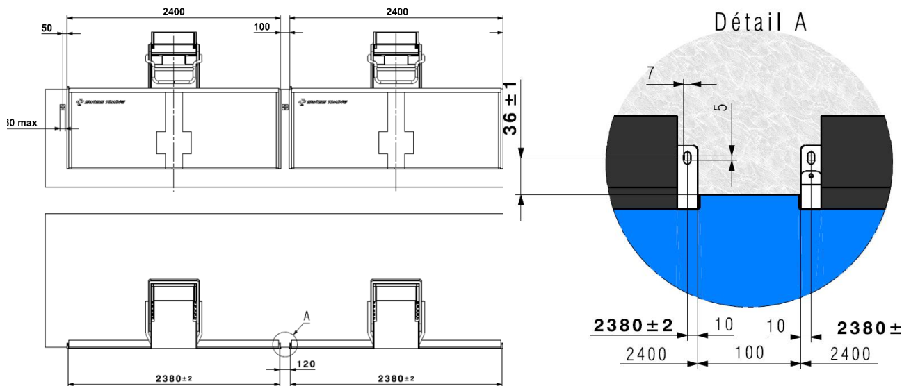
Abbildung 5 - Anschlagplatte 240x90 / Befestigung ohne Haltewinkel
