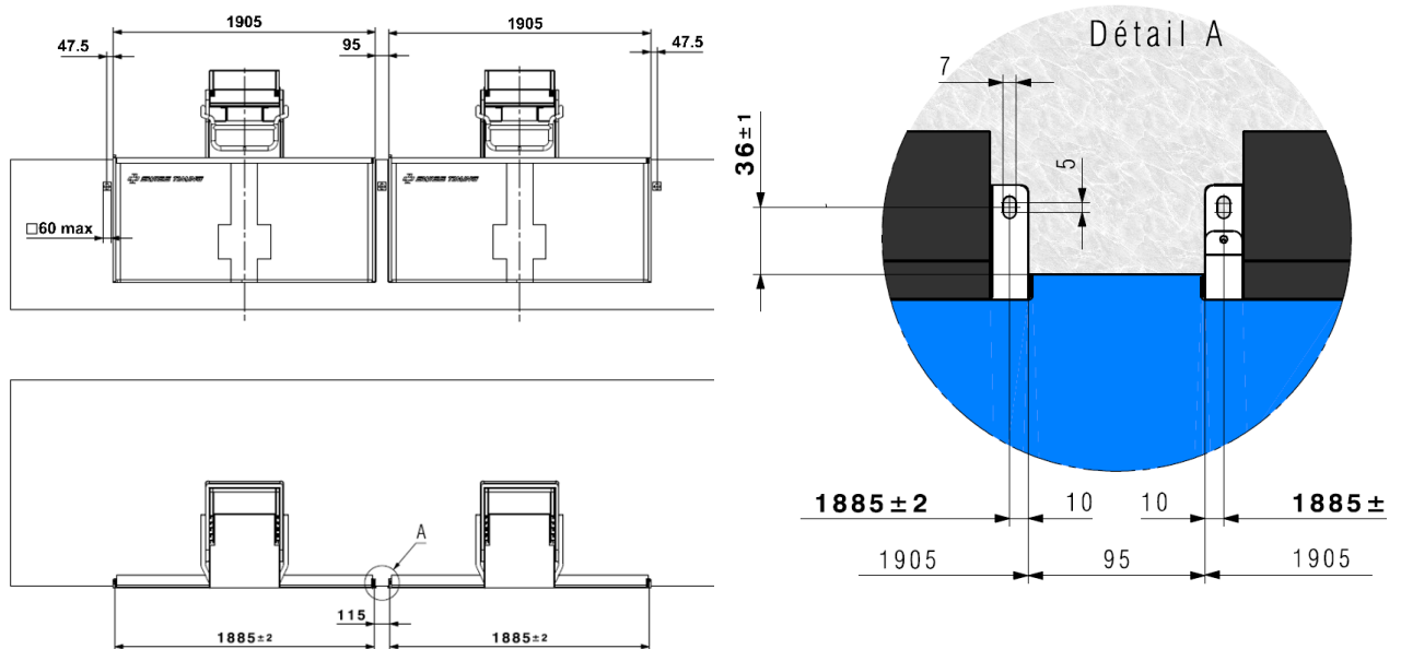
Abbildung 7 - Anschlagplatte 190x90 / Befestigung ohne Haltewinkel
