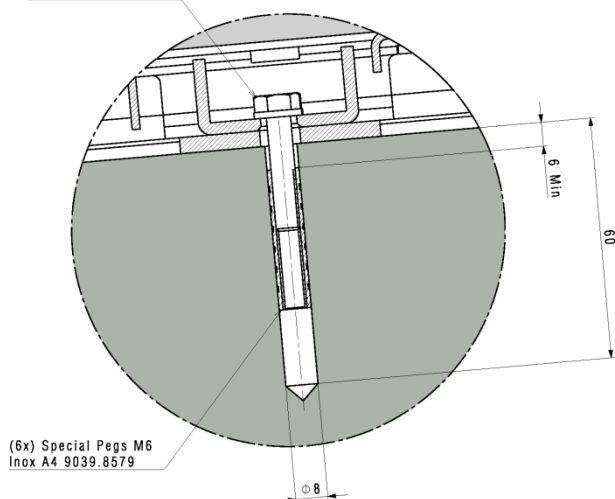
Détail C
